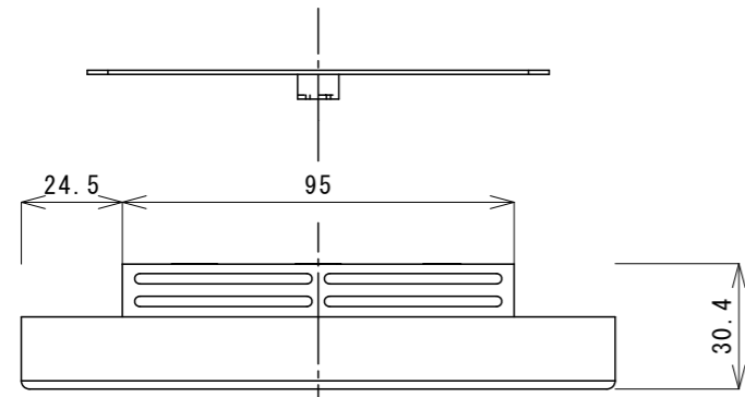
コントローラ上面図
