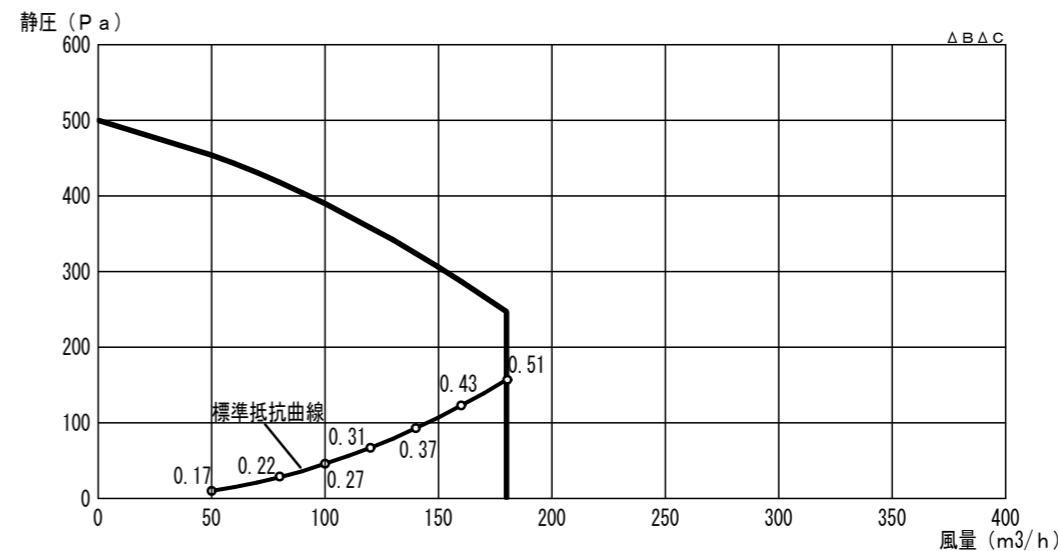
LWZ-70E 給排気 P-Q 特性図 ※○の数値は比消費電力 (W/m³/h)
